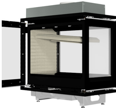
Retrait du premier déflecteur
