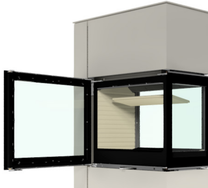
Entfernen Sie das obere Rauchabweisblech
