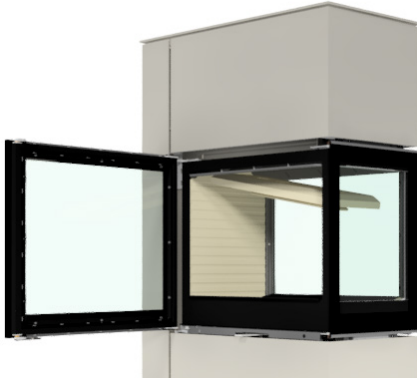
Entfernen Sie die erste Rauchumlenkungsplatte
