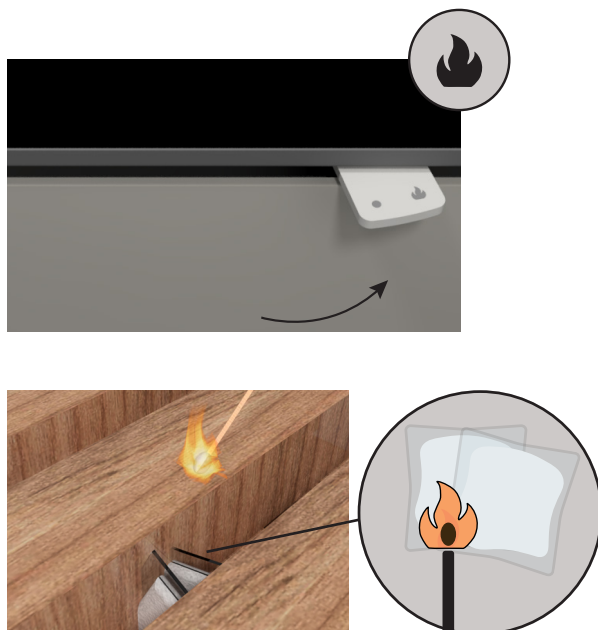
Zündung der Zündungspakete
